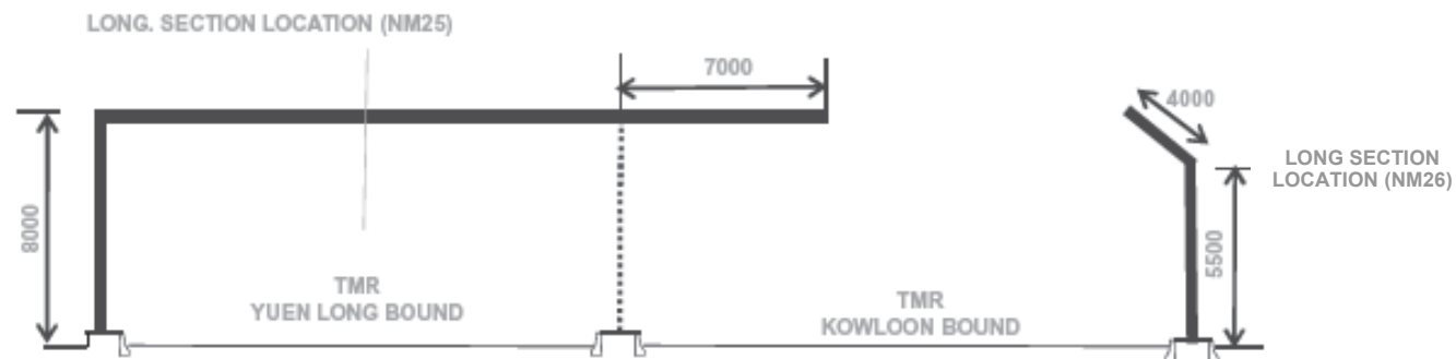
SECTION 16-16 SEMI-ENCLOSURE NM 25 & BARRIER NM 26 (N.T.S.)
